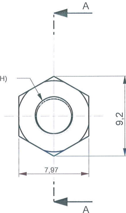
ELEVATION
